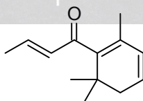
beta-damascenone
